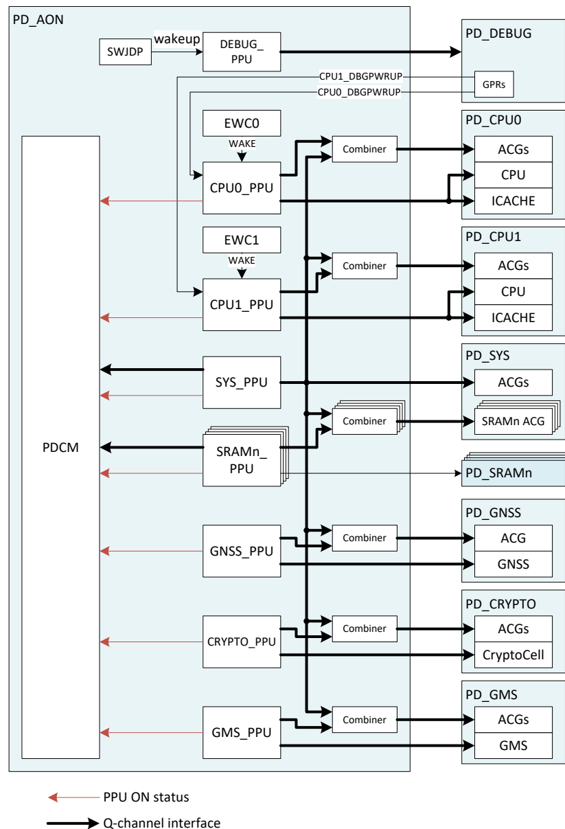
Рисунок 2.8. Схема взаимодействия РРУ
