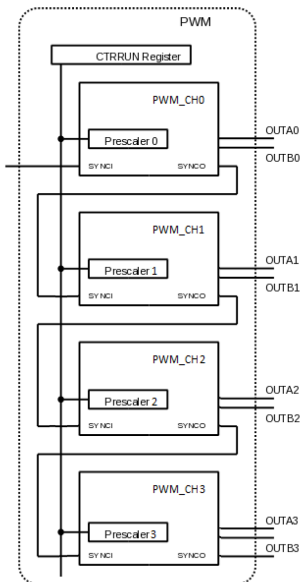
Рисунок 17.4. Управление пуском предделителей различных каналов PWM
