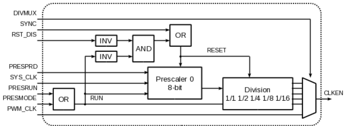
Рисунок 17.3. Функциональная схема предделителя частоты
