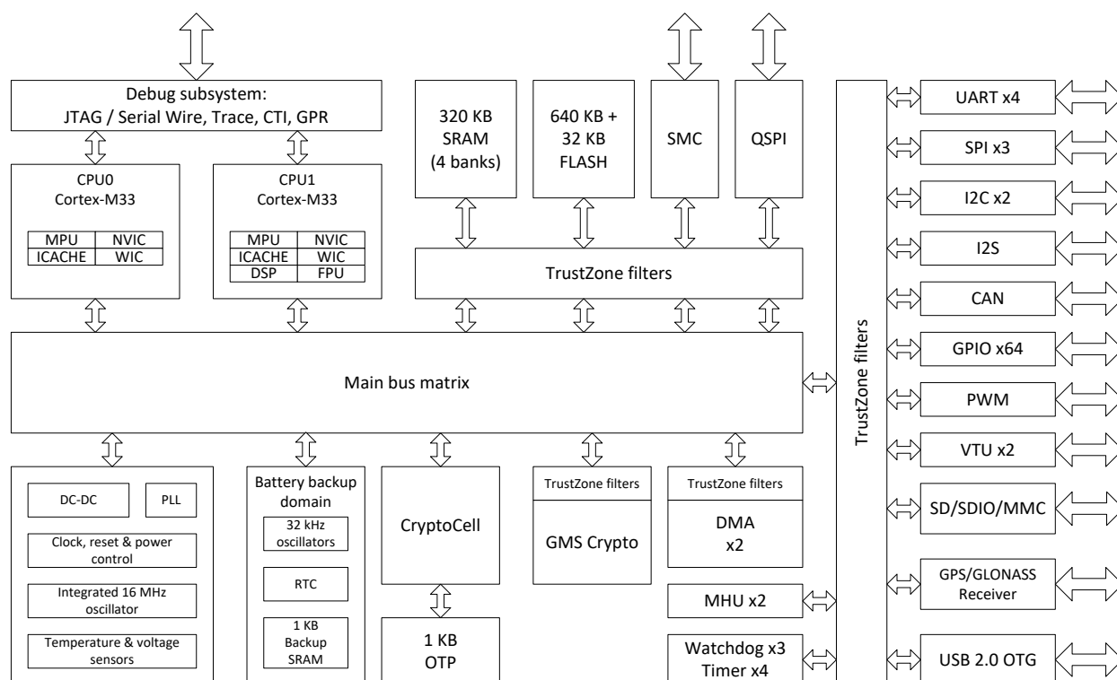
Рисунок 1.1. Блок-схема K1892ВГ1Я
