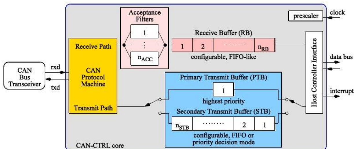
Рисунок 15.2. Концепция буферов сообщений
