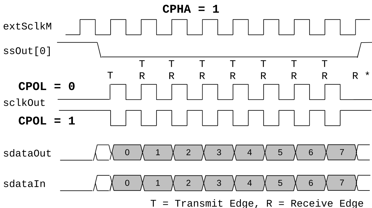
Рисунок 18.5. Передача данных Master-устройства SPI при CPHA = 1, CPOL = 0, 1
